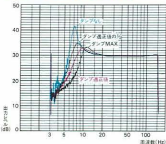
●エレクトロ・ダイナミック・サーボ・トーンアームのfo、Qダンプ特性 可聴周波数域には影響をあたえずに超低域の鋭いピークを制動することができます。
