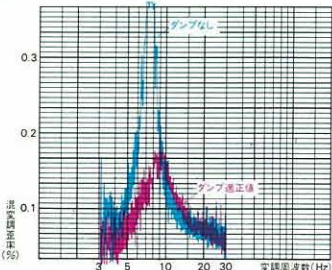
図⑤ 混変調波形比較
