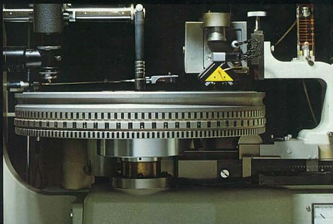
クォーツロック・カッティング・システム(ビクター 青山カッティング・センター)
