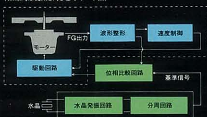
クォーツロック・サーボ・システムの基本ブロック・ダイアグラム (点線内は従来と同じ基本サーボ系)
