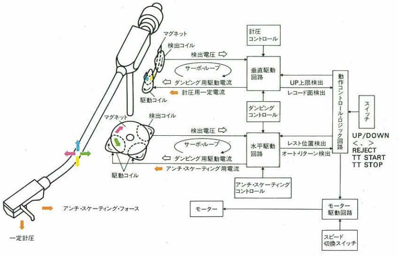
●ダブル・ダイレクト・ドライブ方式 エレクトロ・ダイナミック・サーボ・トーンアームの動作原理図
