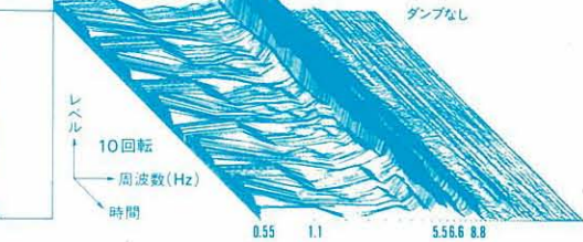
●K&K測定法によるSN比特性比較(無音溝レコード)
