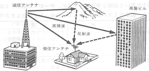
マルチパスの起きる原因
