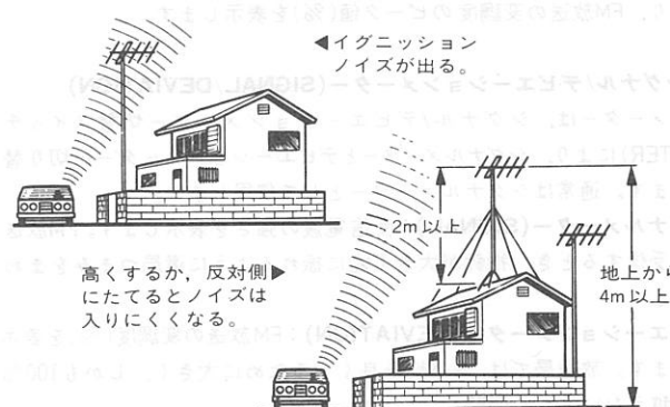
FM専用外部アンテナの設置位置
