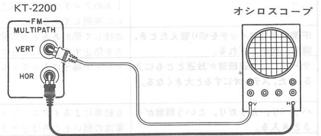
オシロスコープとの接続
