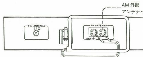
図4 AMリードアンテナの設置
